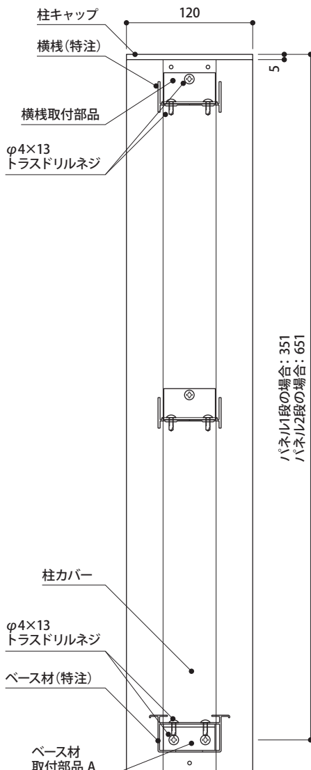
B部詳細図
