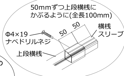
図1-② 横棧スリーブの取付け
