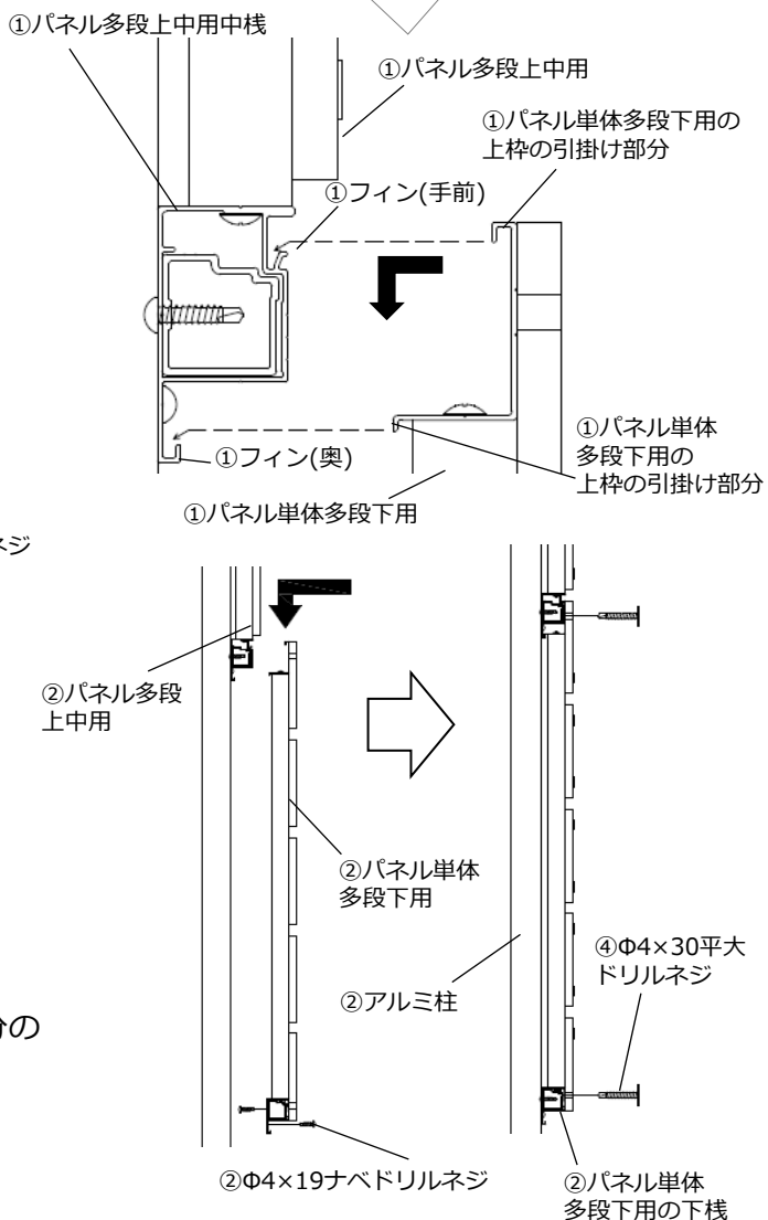
図3-① 中棧へパネル引掛け
