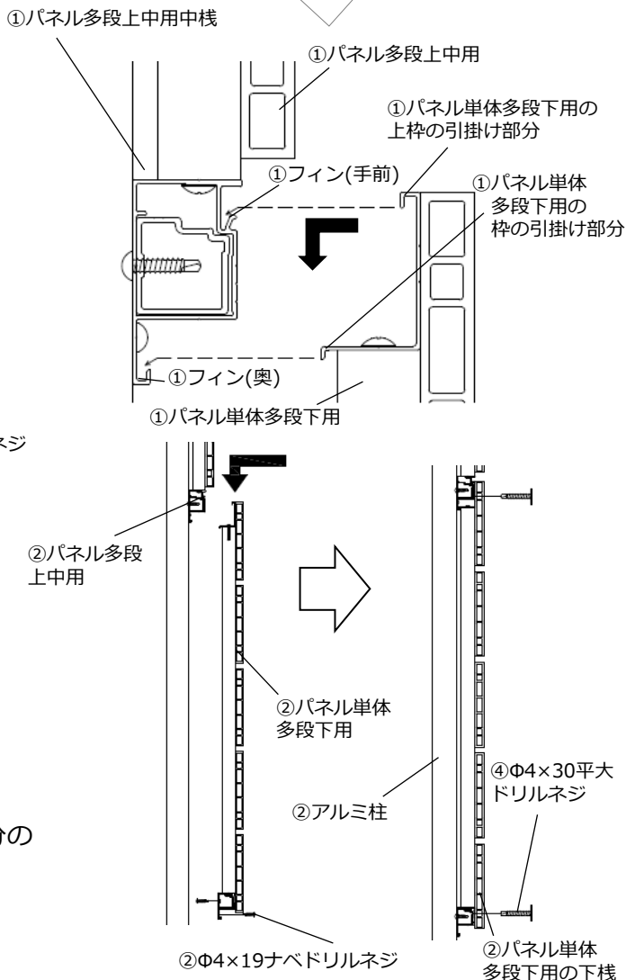
図3-① 中棧へパネル引掛け
