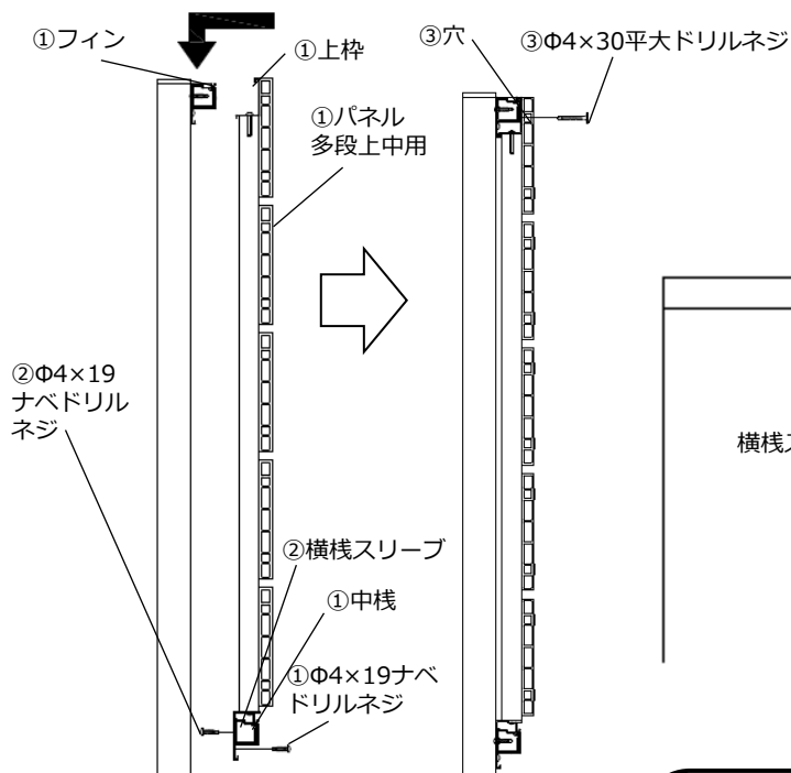
図2-① 上段横棧へのフィンの引掛け
