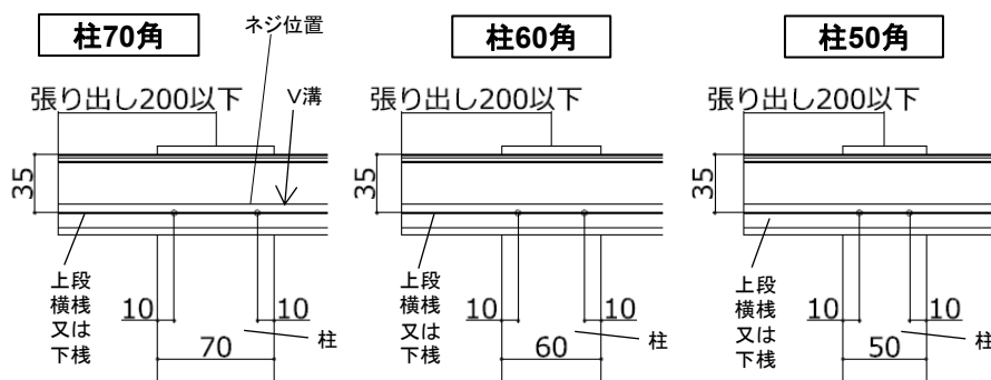
図1-① 上段横棧下棧の柱への取付け
