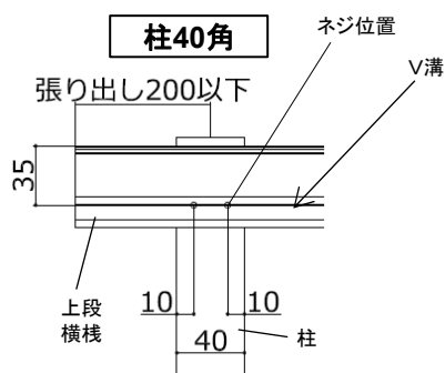
図1-① 上段横棧の柱への取付け
