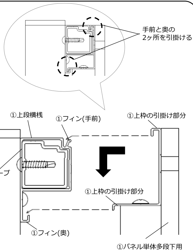
図2-① 上段横棧へのフィンの引掛け
