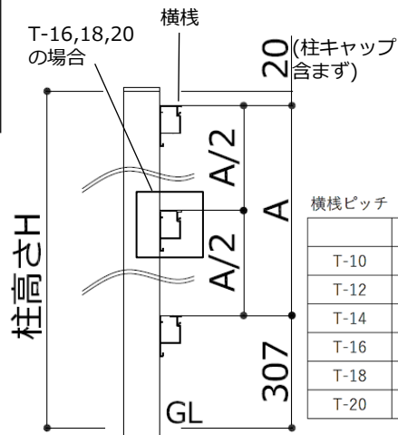
柱横棧納まり図
