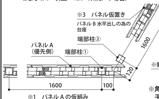
※1 パネルAの仮組み
