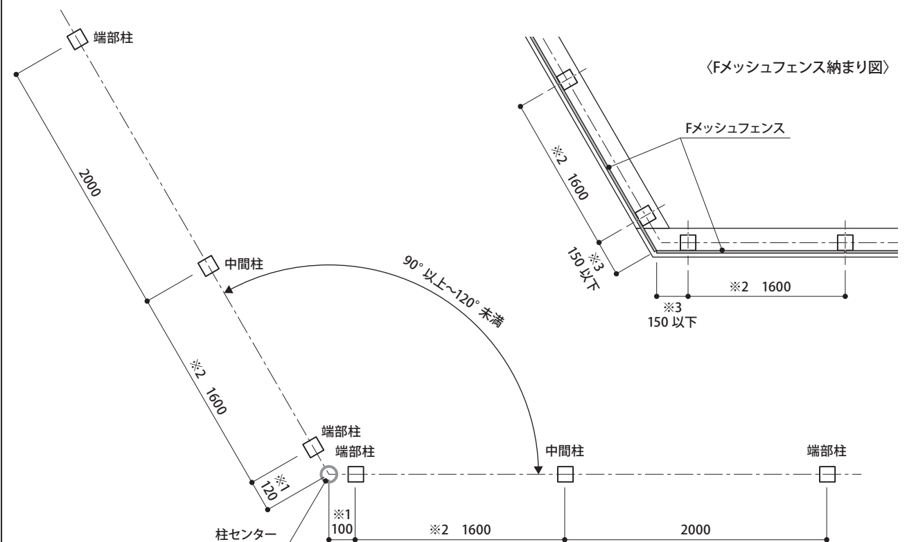
フリーコーナー部 (鈍角)
