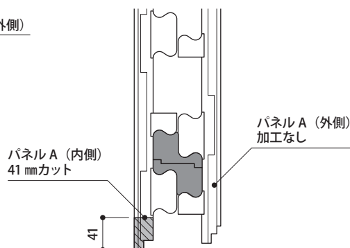
①〈パネルA（内側）加工図〉
