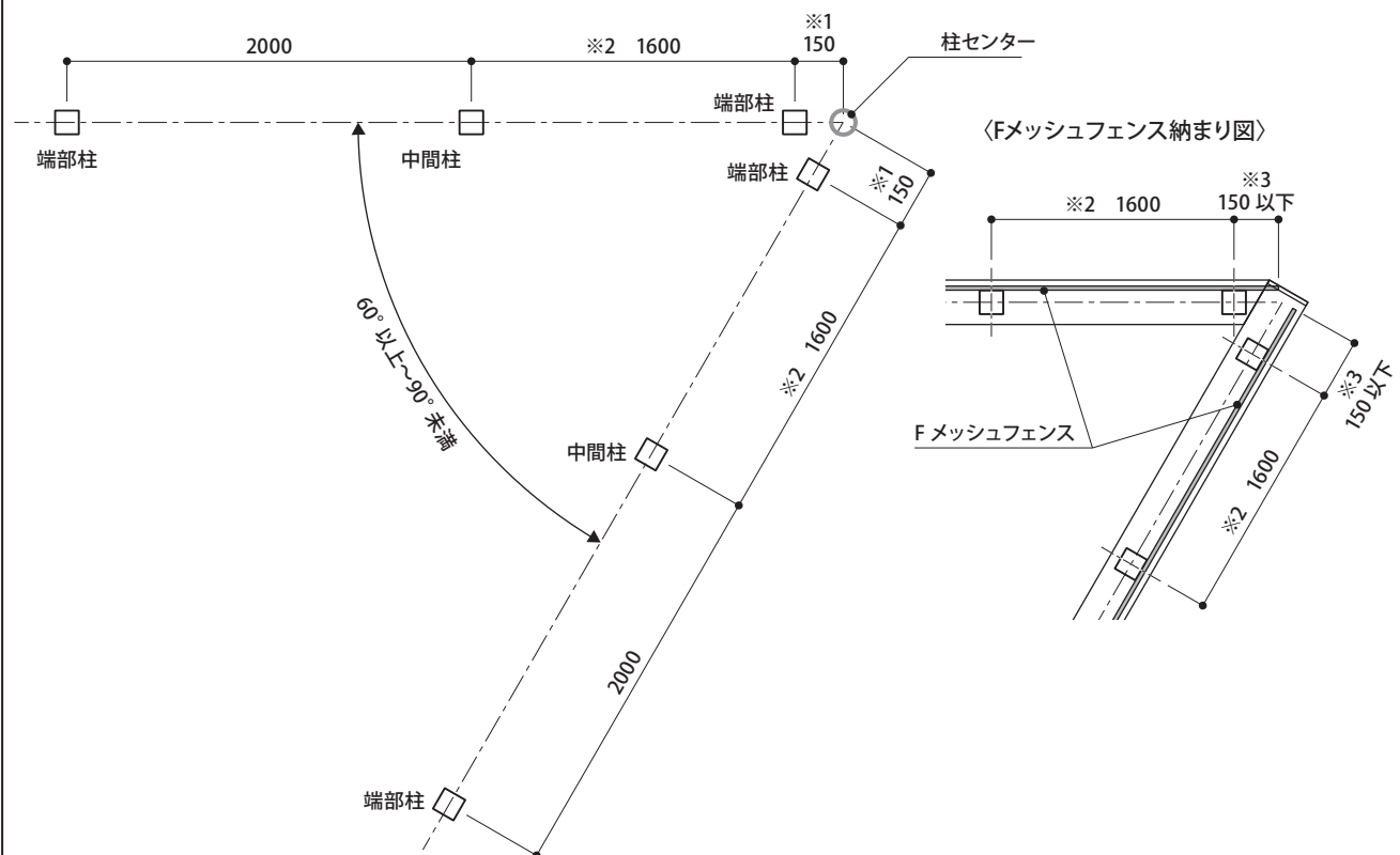
フリーコーナー部 (鋭角)
