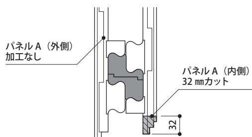
①〈パネルA（内側）加工図〉
