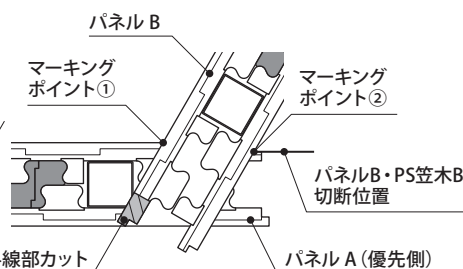
※2 パネルBのマーキング
