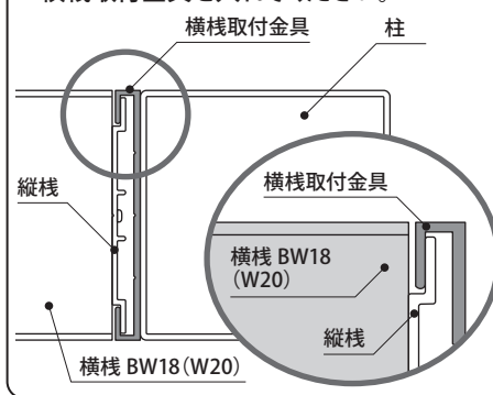
横棧BW18 (W20)・横棧取付金具納まり図
