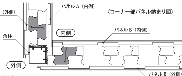
②〈パネルB（内側）加工図〉
