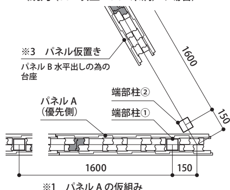
※1 パネルAの仮組み
