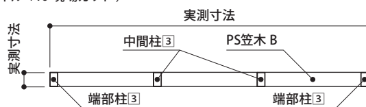
PS 笠木カバー (アクセントパネル+10 現場カット)
