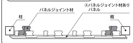
(A)パネルジョイント材ありパネル納まり図
