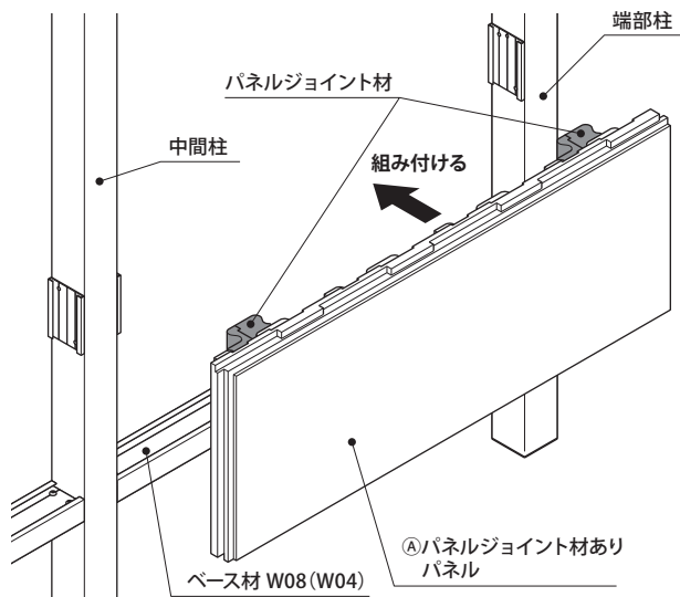
(A)パネルジョイント材ありパネル納まり図
