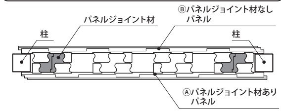
(A)パネルジョイント材あり・(B)パネルジョイント材なしパネル納まり図
