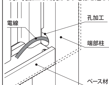
A部拡大図
