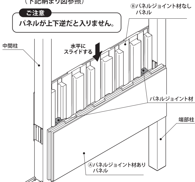
(A)パネルジョイント材あり・(B)パネルジョイント材なしパネル納まり図
