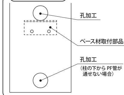
柱配線用加工図
