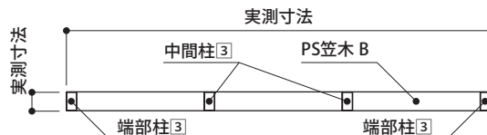
PS 笠木カバー (アクセントパネル +10 現場カット)
