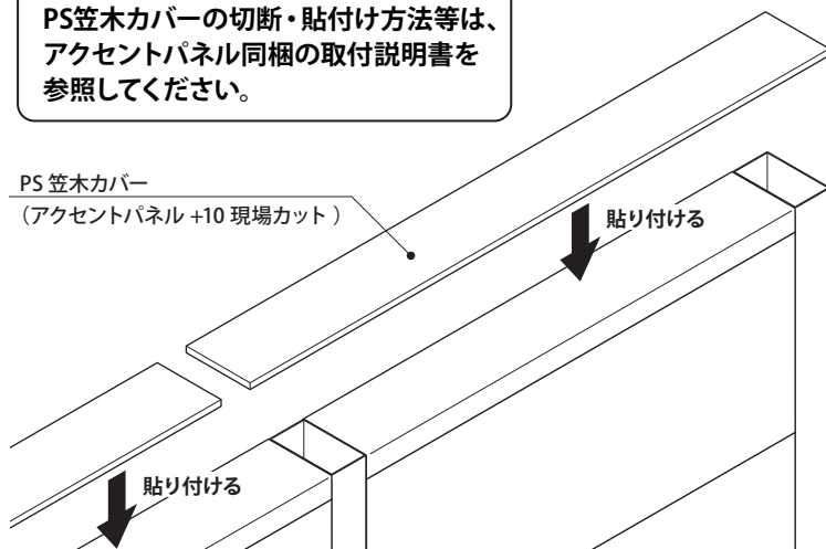
PS 笠木カバー (アクセントパネル +10 現場カット)
