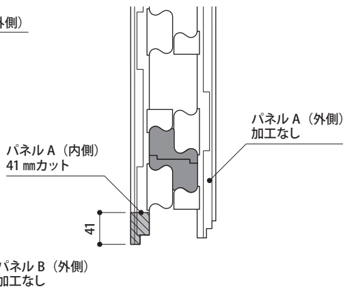
①〈パネルA（内側）加工図〉
