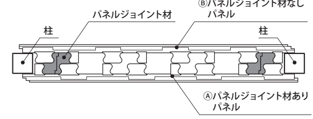
(A)パネルジョイント材あり・(B)パネルジョイント材なしパネル納まり図
