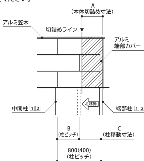
本図は、アルミ笠木・アルミ端部カバー仕様
