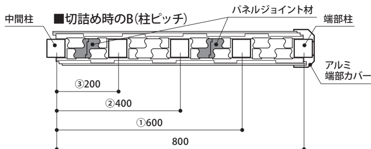
本図はパネルW08の場合です。
