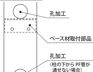
柱配線用加工図
