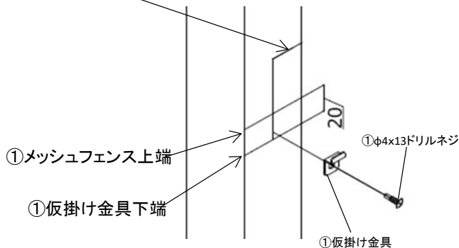
フェンス2段仕様の場合
