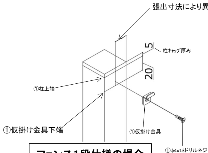
フェンス1段仕様の場合
