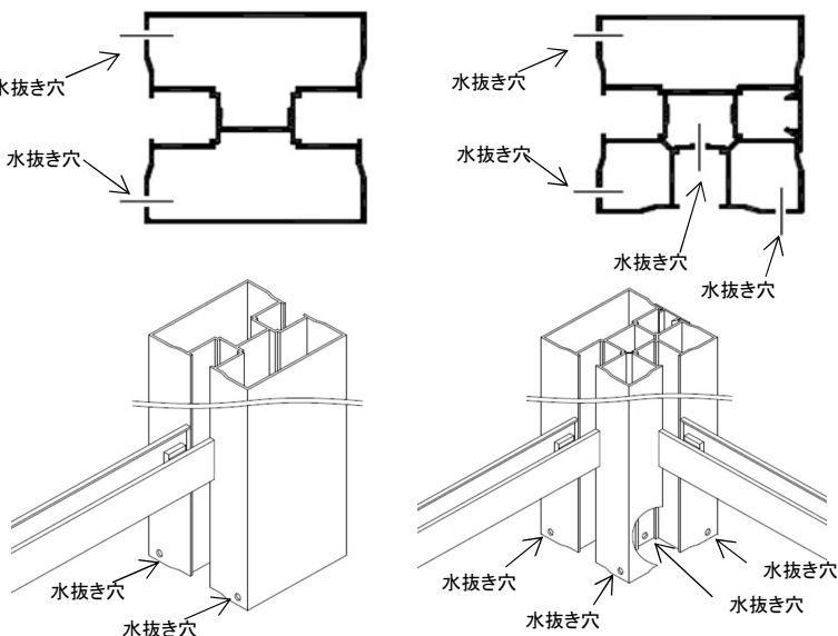
中間・端部柱
