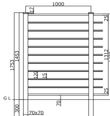
板10段 (T-14)
