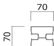
中間柱
