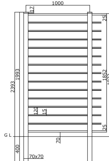
板14段 (T-20)
