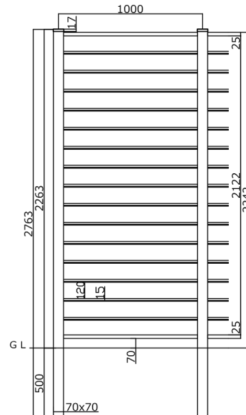
板16段 (T-22)
