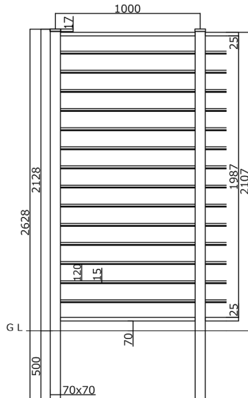
板15段 (T-21)
