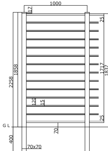
板13段 (T-18)
