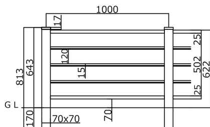
板4段 (T-6)
