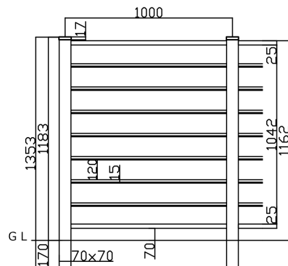
板8段 (T-12)
