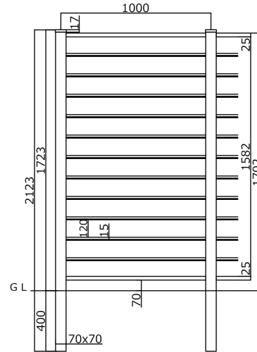
板12段 (T-17)
