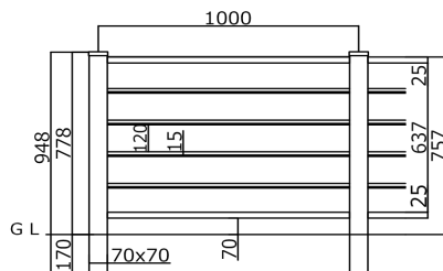
板5段 (T-8)
