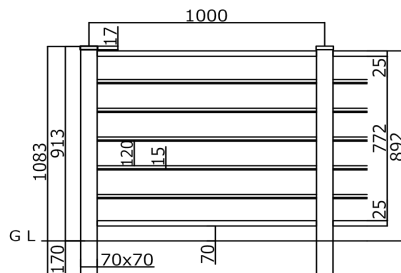
板6段 (T-9)
