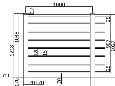
板7段 (T-10)
