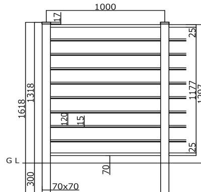
板9段 (T-13)
