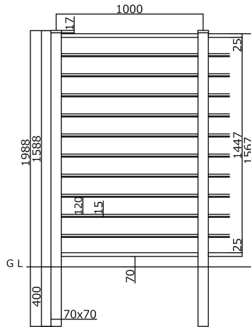
板11段 (T-16)
