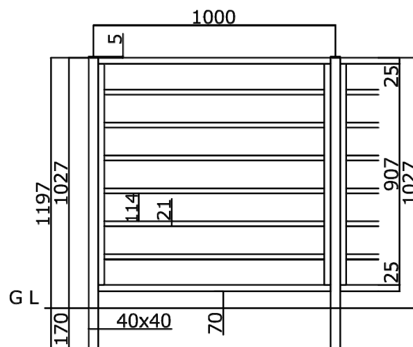
板7段 (T-10)
