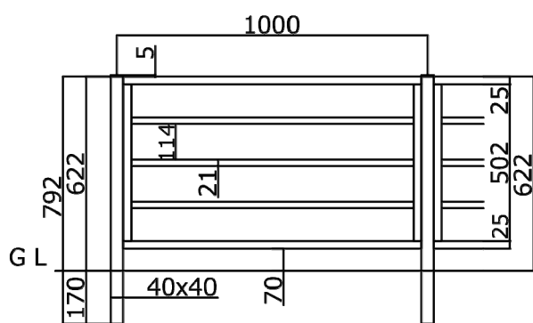
板4段 (T-6)
