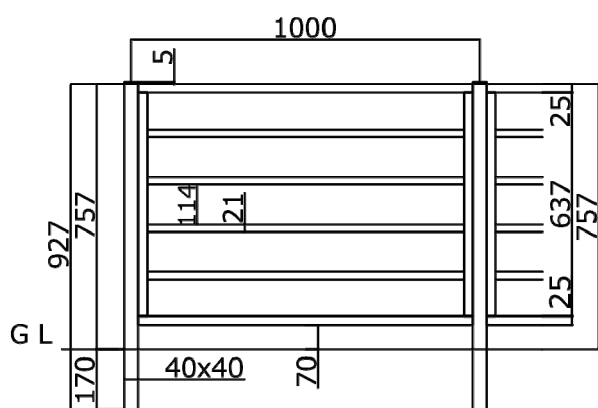
板5段 (T-8)
