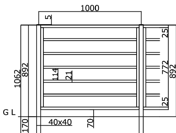
板6段 (T-9)
