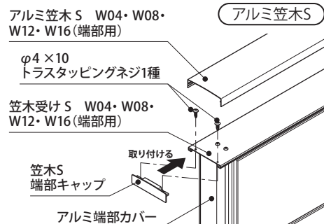
●アルミ笠木Sの取り付け
