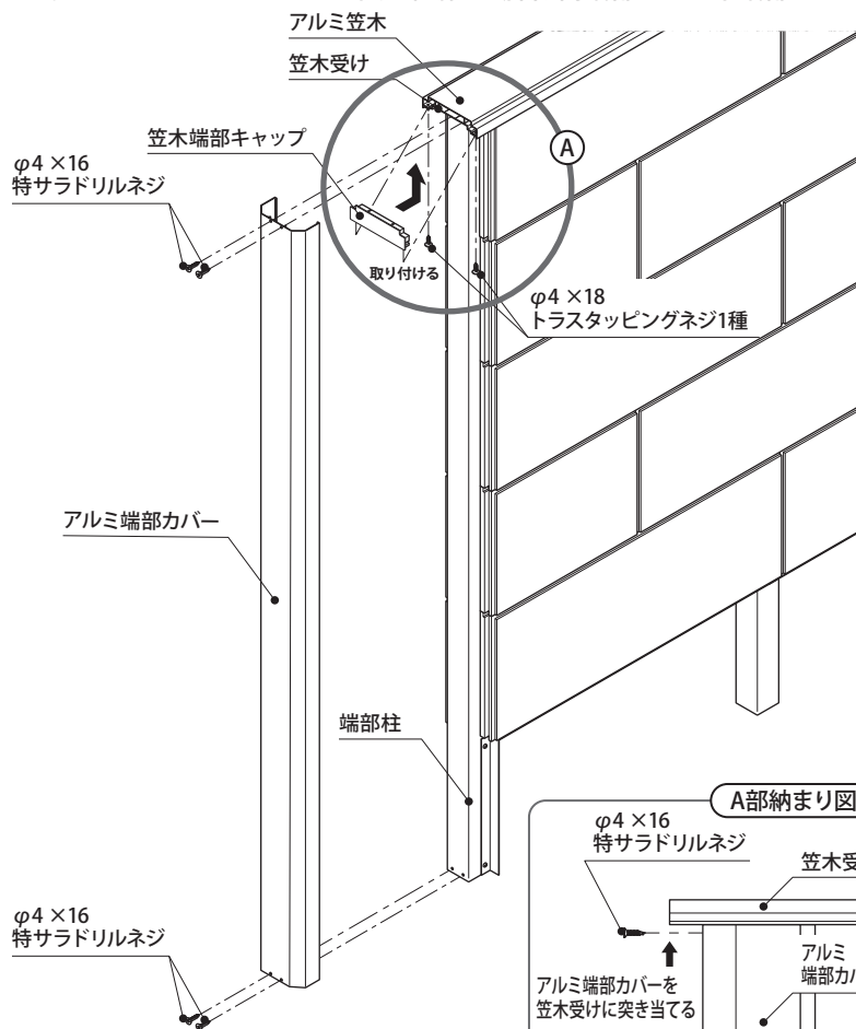
●アルミ笠木Sの取り付け
