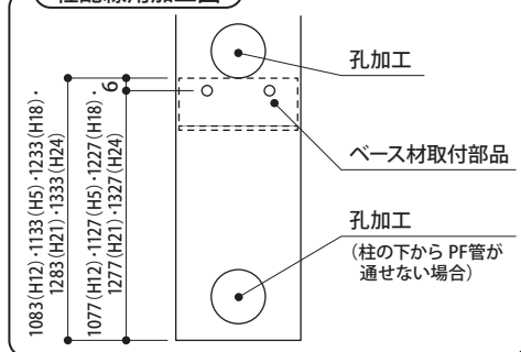
柱配線用加工図
